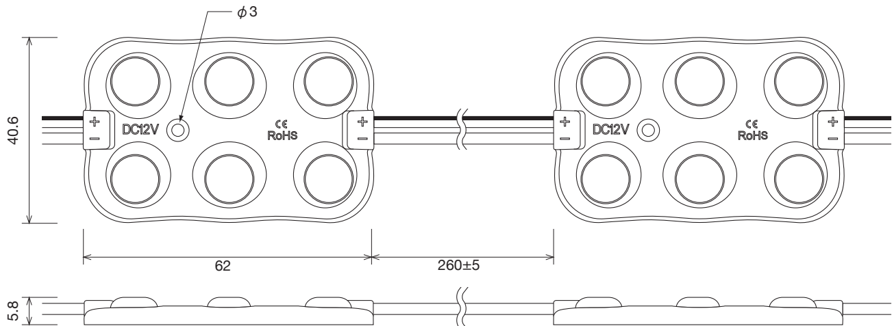
製品寸法図 (mm)
